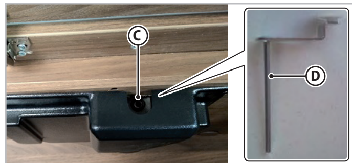
Rys. 6.20 - Elektryczne odblokowanie łóżka typu A
