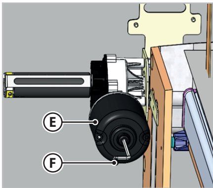
Rys. 6.21 - Elektryczne odblokowanie tóżka typu B
