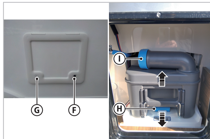
Rys. 6.45 - Opróżnianie kasety WC
