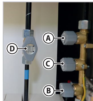
Rys. 6.27 - Zawory dystrybucji gazu
