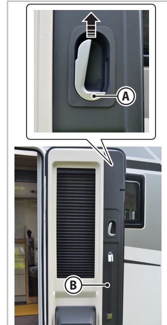
Rys. 5.2 - Otwieranie/zamykanie drzwi wejściowych od wewnątrz
