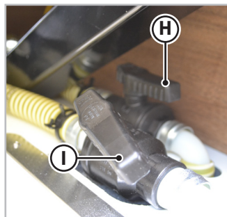
Rys. 6.39 - Zawór opróżniania czystej wody w podłodze podwieszanej
