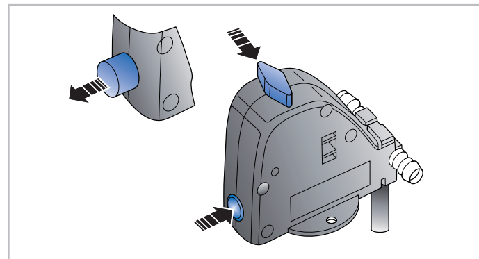
Rys. 6.47 - Zawór bezpieczeństwa grzejnika Combi
