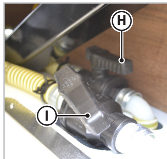
Fig. 6.39 - Tømmeventil for rentvannstanken dobbelt gulv
