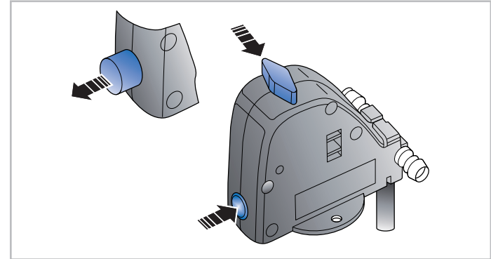
Fig. 6.47 - Kombi-sikkerhetsventil
