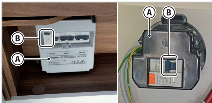
Sl. 6.32 - Razvodna ploča
