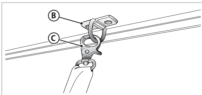
Sl. 6.23 - Kuka za sigurnosnu mrežu
