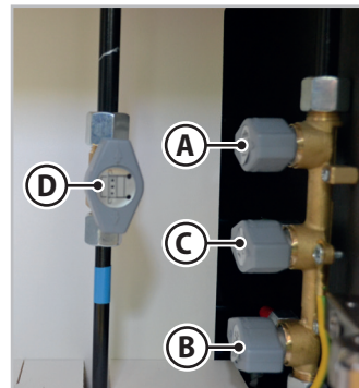
Sl. 6.27 - Slavine razdjelnika plina
