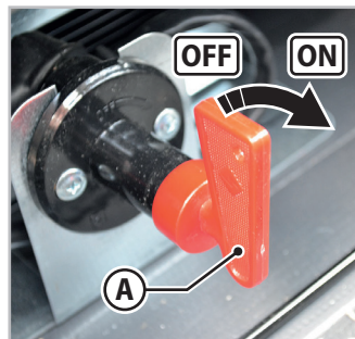
Sl. 6.35 - Prekidač za isključivanje akumulatora
