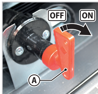
Fig. 6.35 - Coupe-batterie
