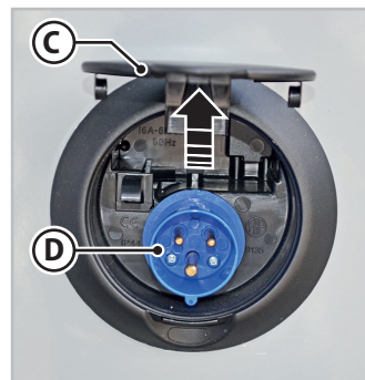
Εικ. 6.33 - Πρίζα τροφοδοσίας 220V
