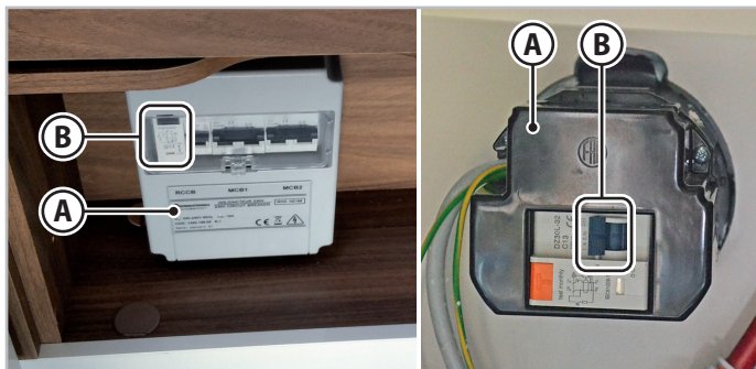
Εικ. 6.32 - Πίνακας τροφοδοσίας
