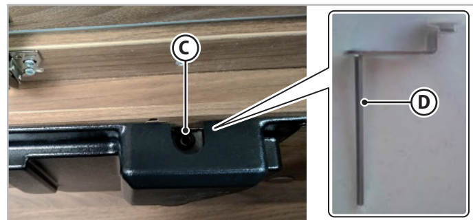
Εικ. 6.20 - Ηλεκτρικό ξεκλείδωμα κρεβατιού τύπου Α
