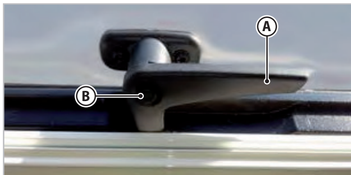
Εικ. 6.2 - Μοχλός κλειδώματος παραθύρων τύπου 1
