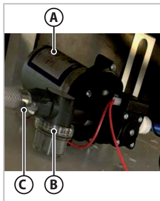
Eik. 7.1 - Εξωτερικό φίλτρο αντλίας νερού
