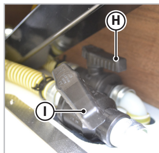
Eik. 6.39 - Βαλβίδα αποστράγγισης καθαρού νερού διπλό δάπεδο
