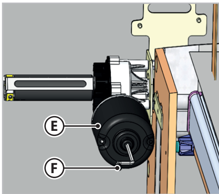
Εικ. 6.21 - Ηλεκτρικό ξεκλείδωμα κρεβατιού τύπου Β
