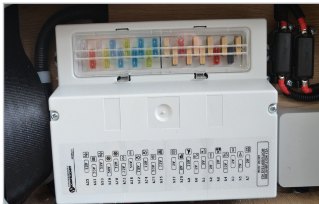
Εικ. 7.3 - Ασφαλειοθήκη με διακόπτη Poliswitch
