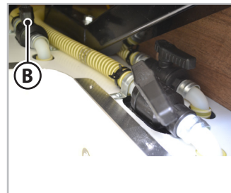
Eik. 6.42 - Βαλβίδα αποστράγγισης βρώμικου νερού διπλό δάπεδο
