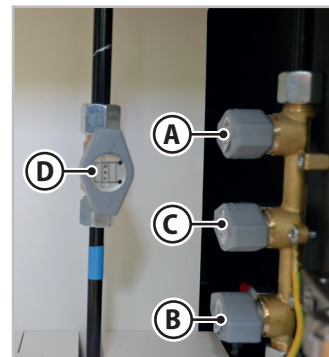
Fig. 6.27 - Gasdistributionens hane
