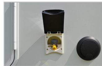
Fig. 6.28 - Udvendigt gasindtag
