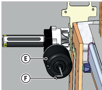
Фиг. 6.21 - Електрическо деблокиране легло тип В
