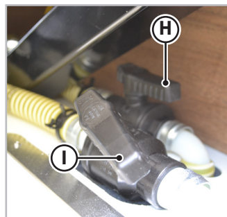
Фиг. 6.39 - Клапан за изпразване на чиста вода с двойно дъно
