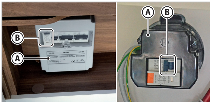
Фиг. 6.32 - Захранващо табло
