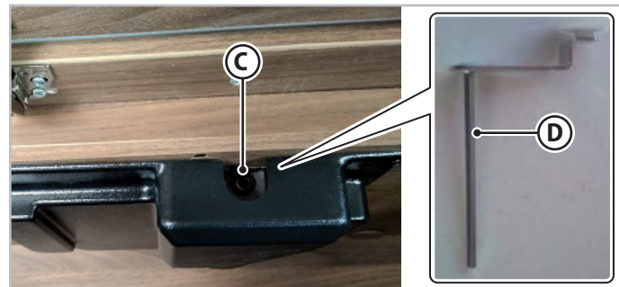
Фиг. 6.20 - Електрическо деблокиране на легло тип А
