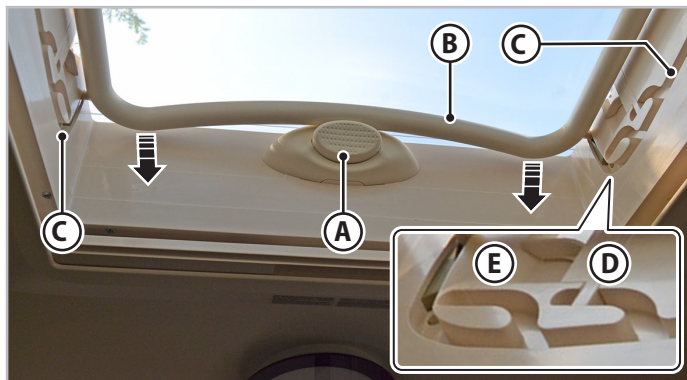
Фиг. 6.10 - Наклянящ се люк - Тип А
