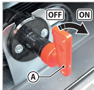
Фиг. 6.35 - Превключвател за изключване на акумулатора
